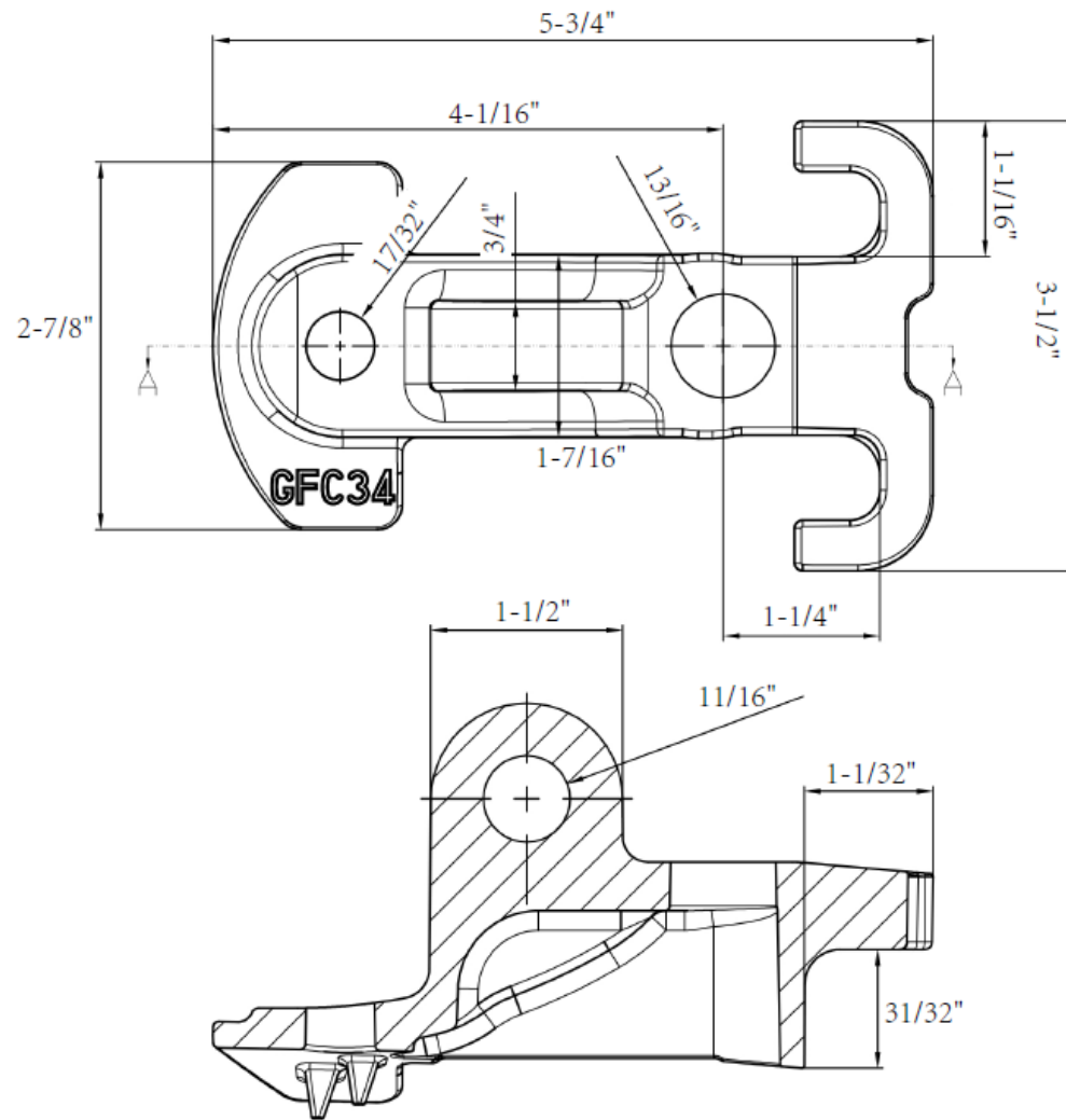
SECTION A-A
